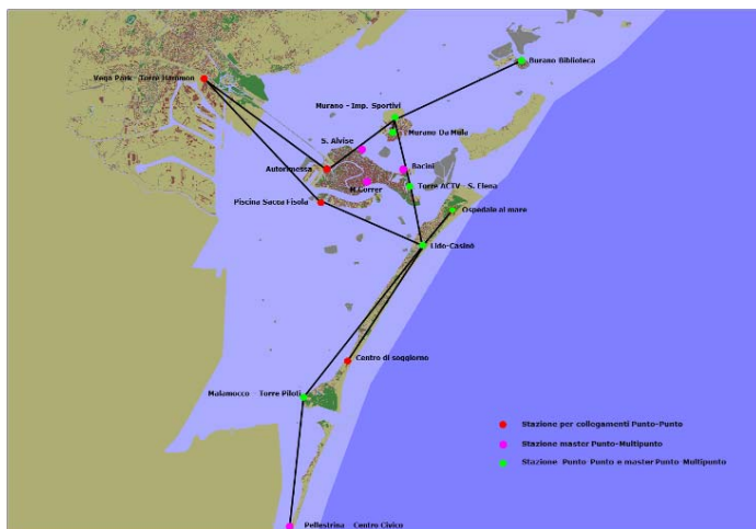
Fig. 3 I ponti radio
